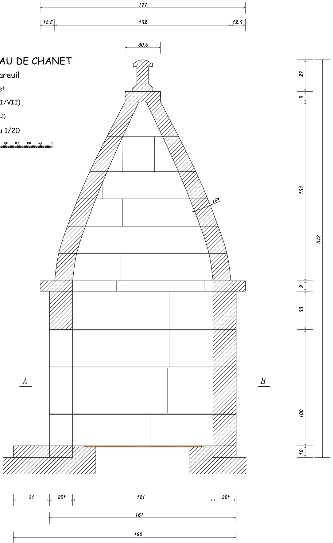
Coupe longitudinale
